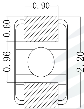
Fig.1-3 Bottom View 背面视图
