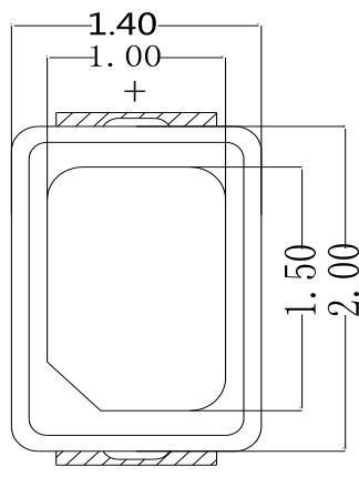
Fig.1-1 Top View 正面视图
