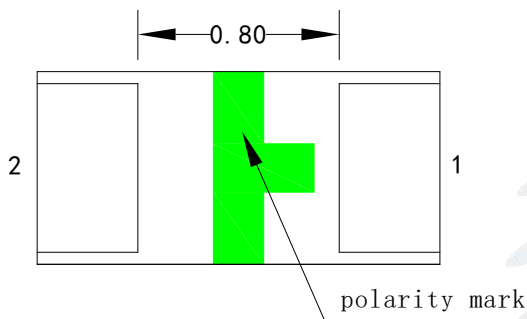
Fig.1-3 Bottom view 背面视图
