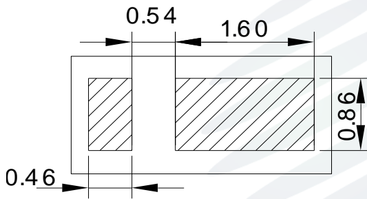
Fig.1-3 Bottom View 背面视图
