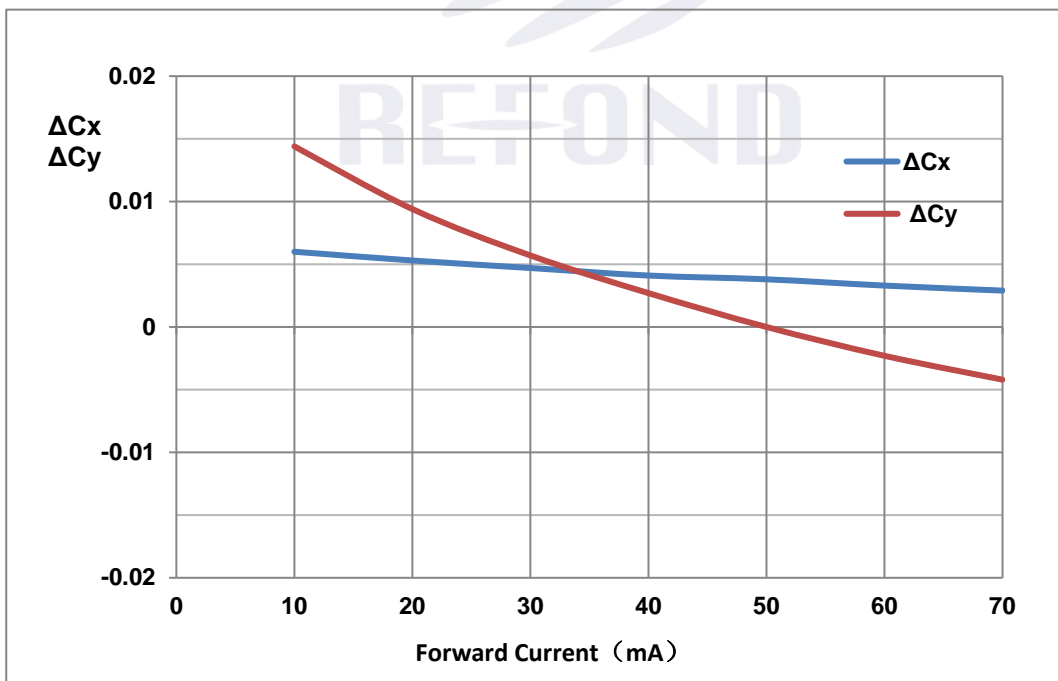
Fig. 1-14 Color coordinate shiftVs Forward Current色坐标偏移与正向电流特性曲线
