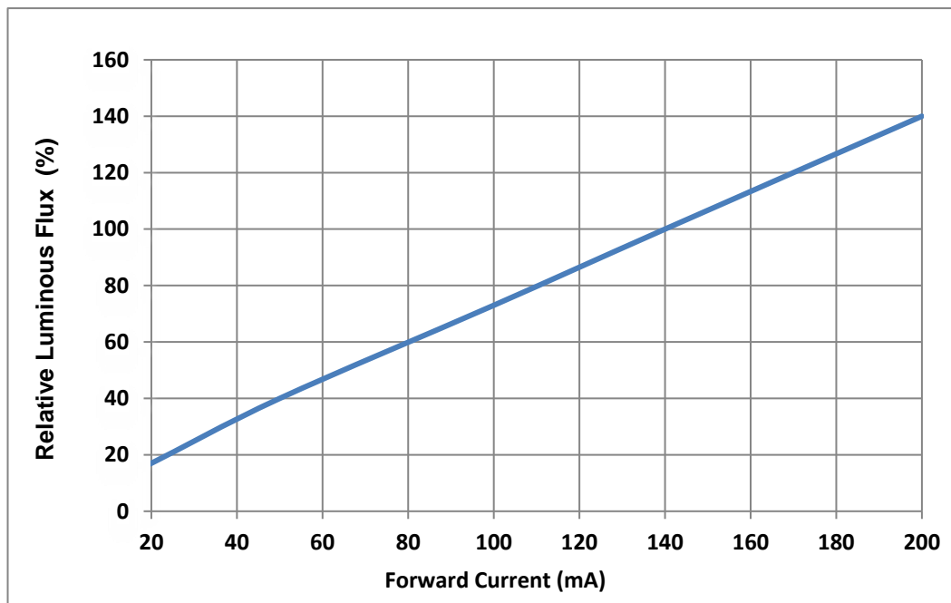
Fig. 1-8 Forward Current Vs Relative Intensity正向电流与相对光通量特性曲线
