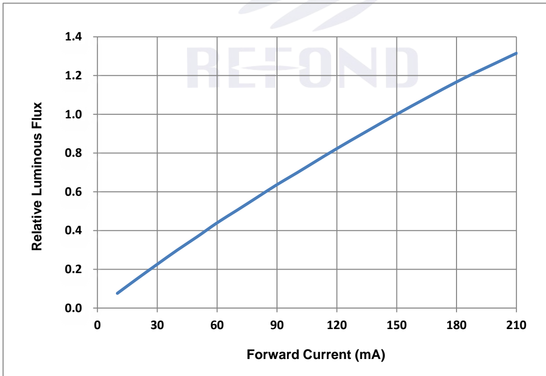
Fig. 1-8 Forward Current Vs Relative Luminous Flux 正向电流与相对光通量特性曲线
