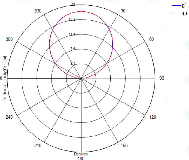
图 10 配光曲线
