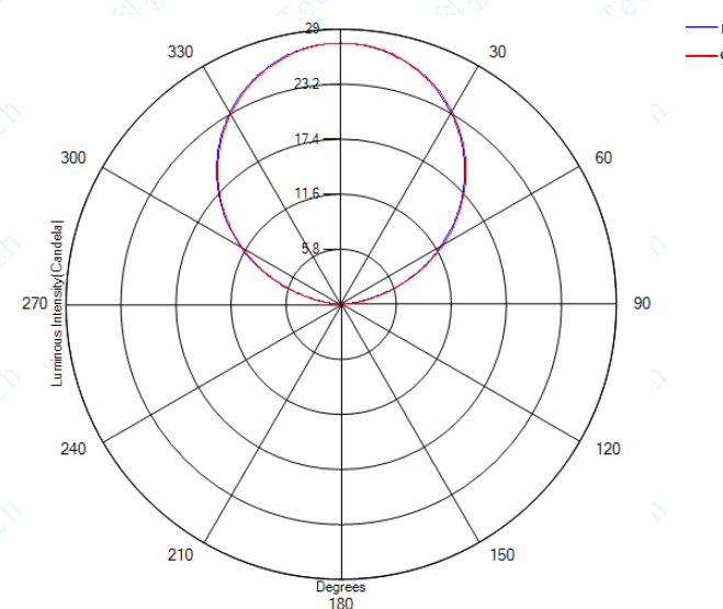
图 10 配光曲线
