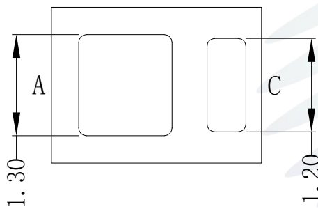
Fig.1-3 Bottom View 背面视图
