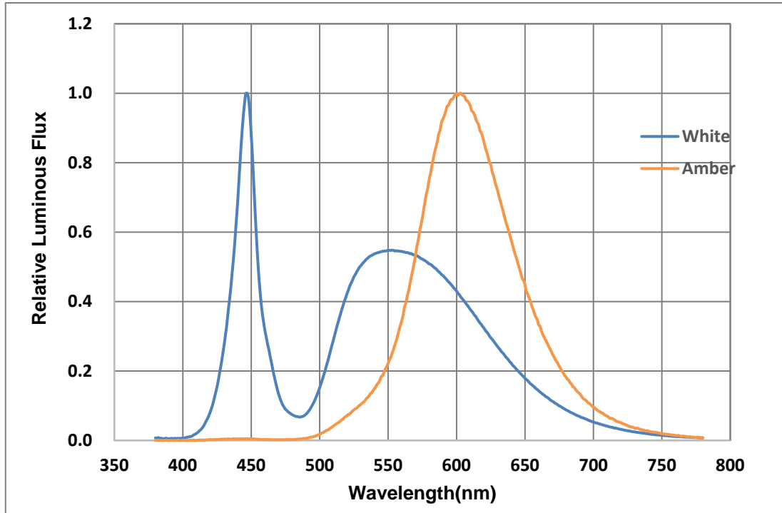
Fig. 1-18 Spectrum Distribution 光谱分布特性曲线
